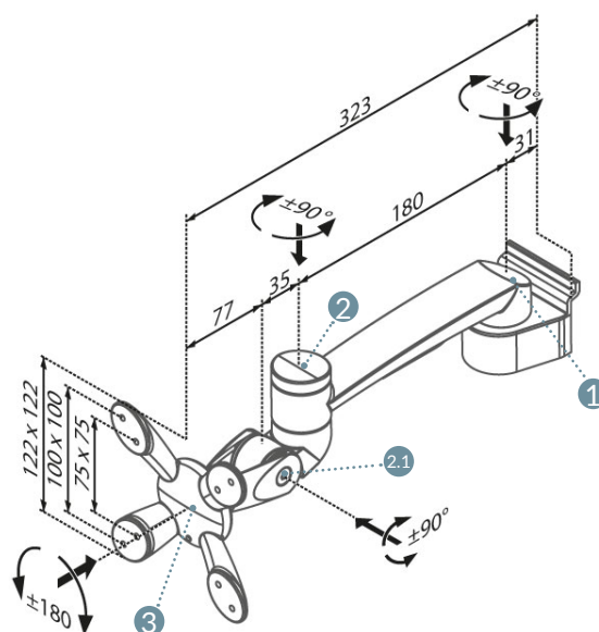
Држач за монитор со 3 зглоба
