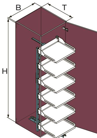
Pleno Standard Систем за вагонетки за високи елементи
