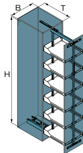
Standard Систем за вагонетки за високи елементи
