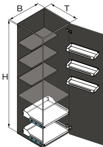
Trio Систем за вагонетки за високи елементи
