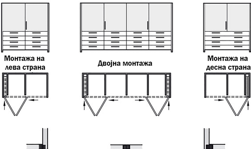
Центрирање на врата со компоненти за магнетно центрирање
