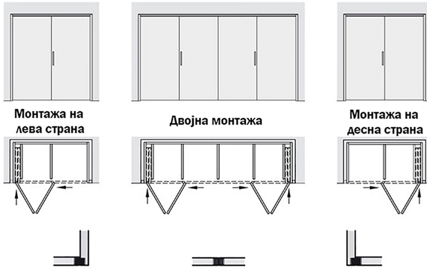
Центрирање на врата со компоненти за магнетно центрирање
