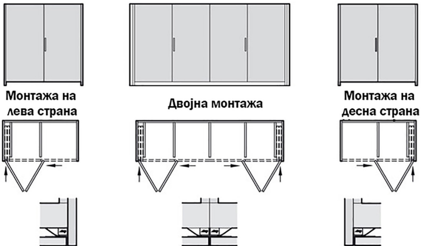
Поставување на рамна врата со внатрешен профил и водечка рампа
