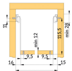
Димензии за Н 150mm
