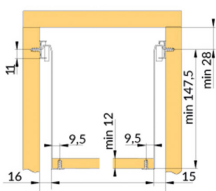
Димензии за Н 150mm
