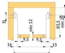
Димензии за Н 118mm
