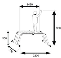
Работна платформа (скеле)
