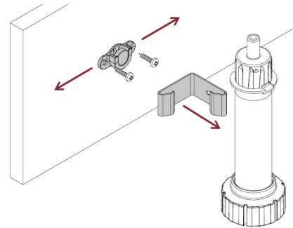
Приказ за монтажа на магнетен држач за цокла од плочест материјал.
