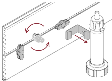
Приказ за монтажа на магнетен држач за пластична цокла.
