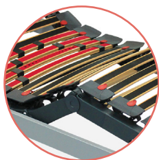
Механизам - предел за подигнување кај нозете
