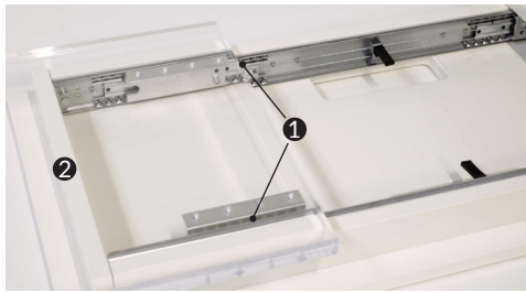
1. Механизам за маса. 2. Рамка за поставување на механизмот.
